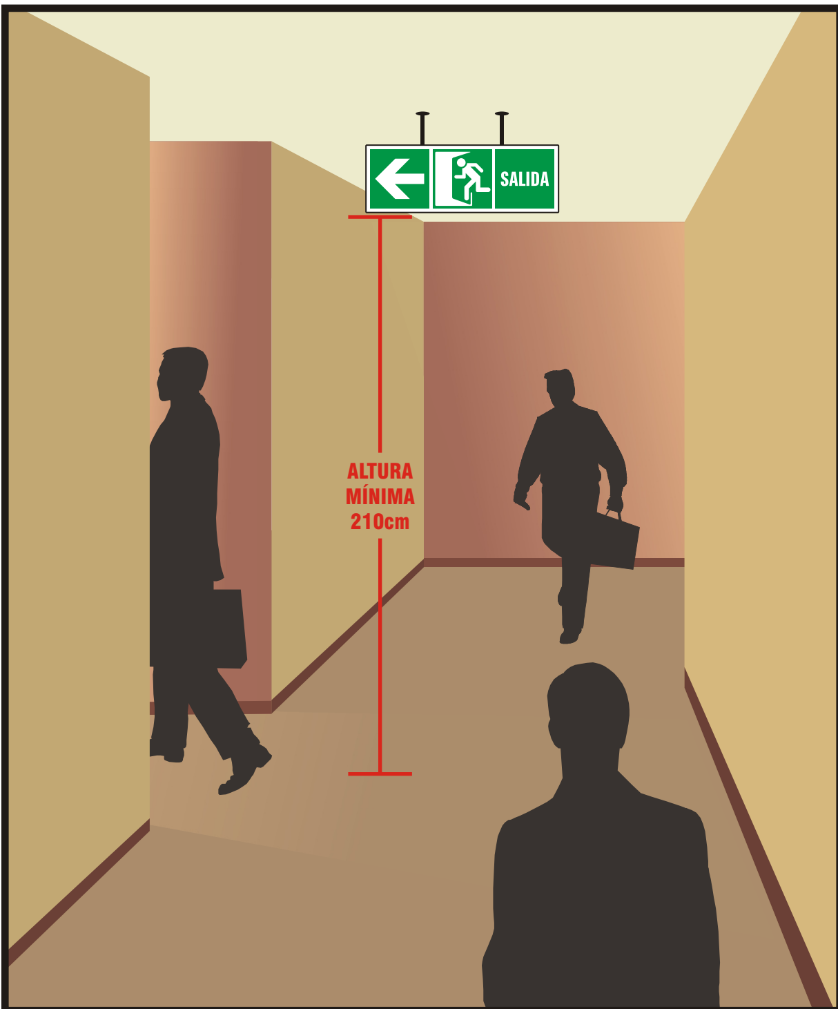
DIBUJO 2 - INSTALACIÓN DE CARTEL DE EVACUACIÓN (TIPO COLGANTE)
